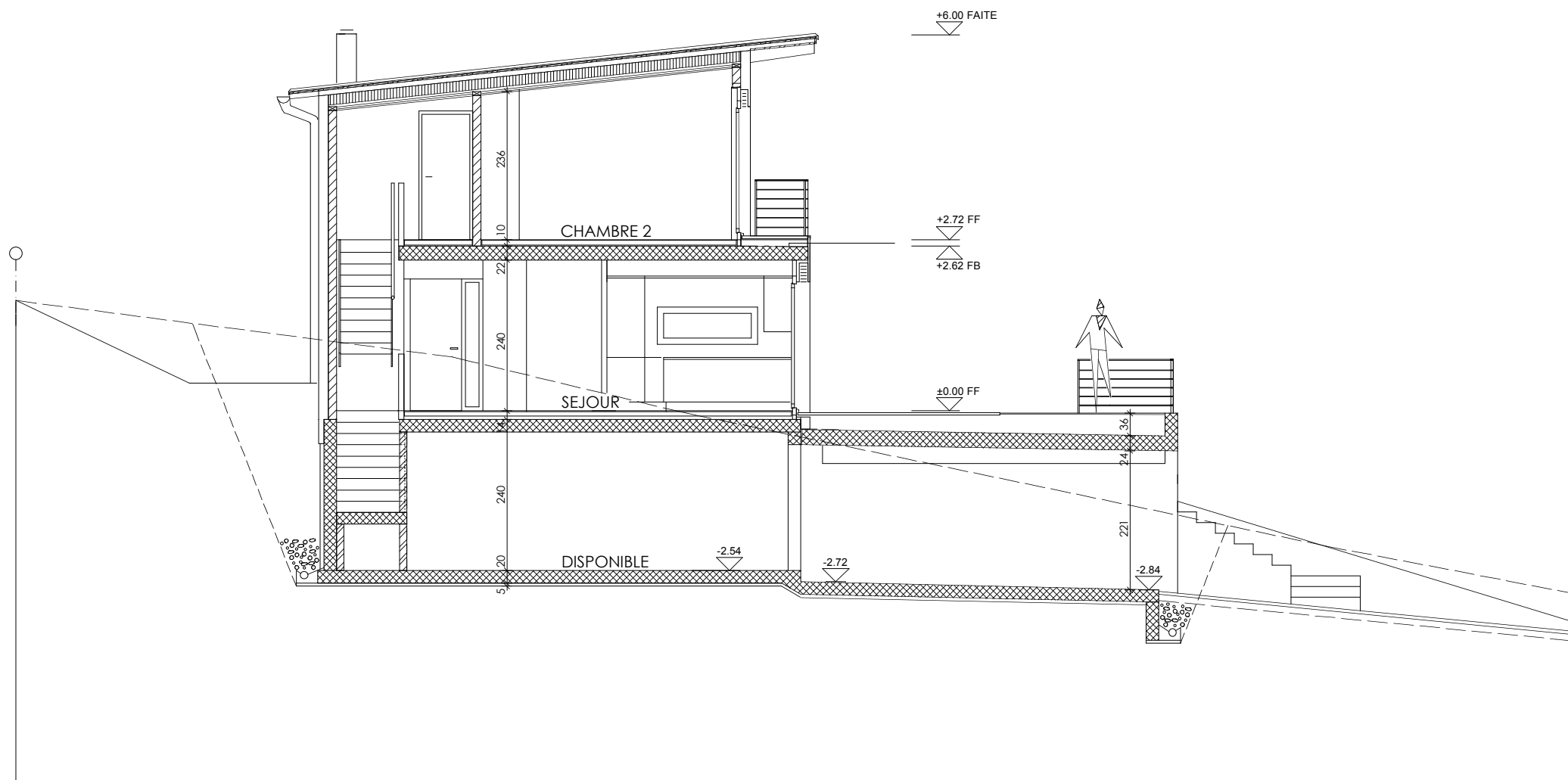
C O U P E A - A
